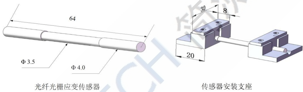
图 2.2 光纤光栅传感器封装形式及传感器安装支座
